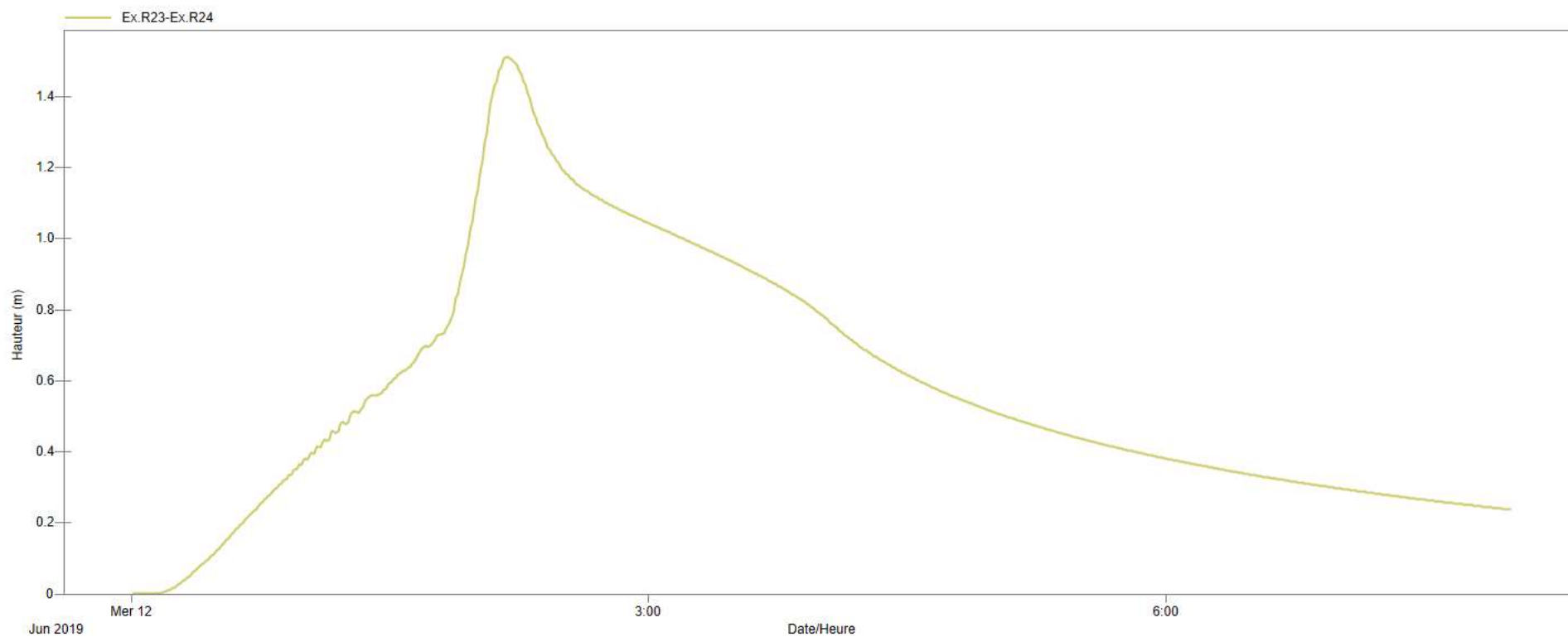
Hauteur d'eau en aval de OD1, au niveau de 1800 existant
